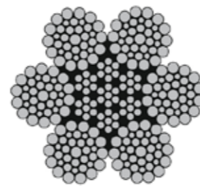
6x36 IWRC
