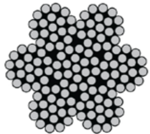
7x19
