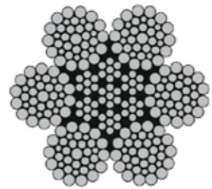
6x36 IWRC
